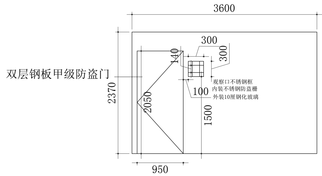
新砌墙剖面 SC=1:50mm
